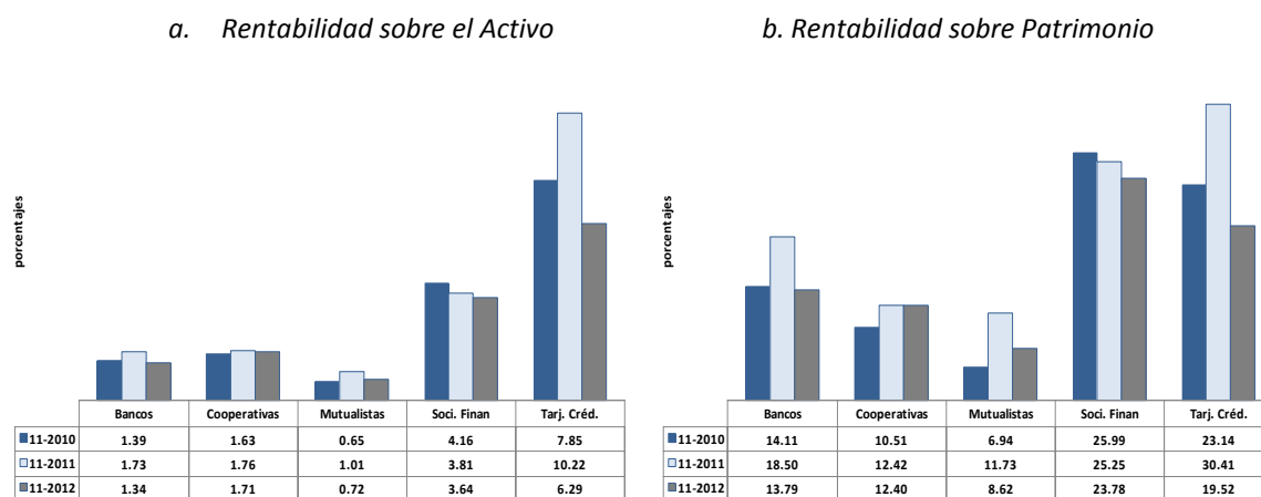
Gráfico 4 SOLIDEZ FINANCIERA MEDIDA POR LA RENTABILIDAD POR TIPO DE SISTEMAS (Porcentajes)
