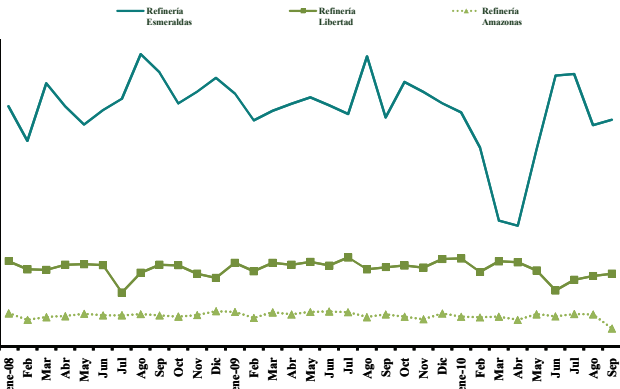
PRODUCCION DE DERIVADOS POR REFINERIAS (miles de barriles)
